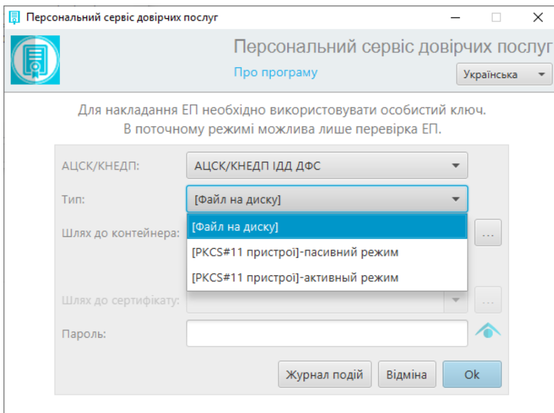
Рис. 27. Вибір Типу для ключового контейнеру
