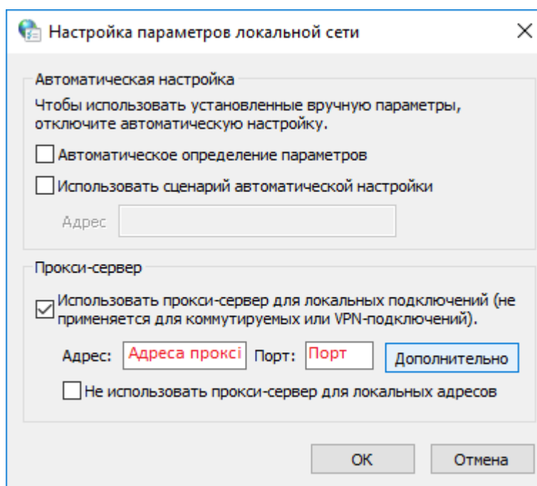
Рис. 7. Налаштування параметрів локальної мережі
