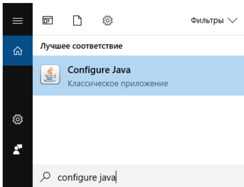
Рис. 9. Конфігурування java-середовища
