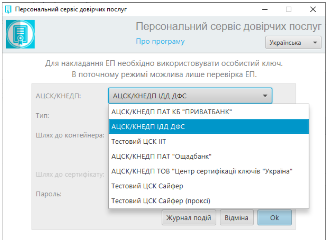
Рис. 26. Вибір КНЕДП/АЦСК
