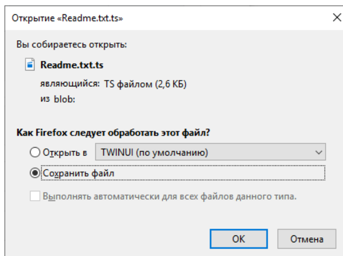
Рис. 75. Збереження файлу
